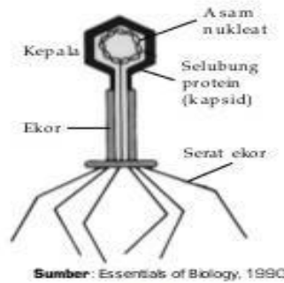
Gambar 2.3 Struktur tubuh virus bakteriofage.
