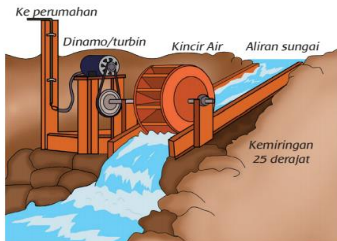
gambar pembangkit tenaga listrik mikrohidro
