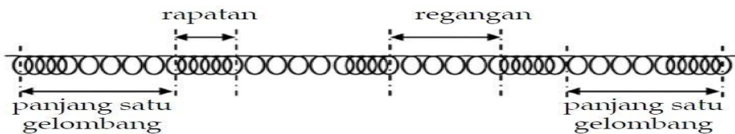
Ilustrasi gelombang longitudinal (Sumber: fisikazone.com)
